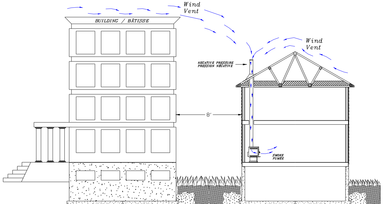
La FIGURE #4 montre bien l'effet de pression négative que peut causer le vent lorsqu'une structure adjacente, telle une bâtisse, est plus haute que la cheminée.
